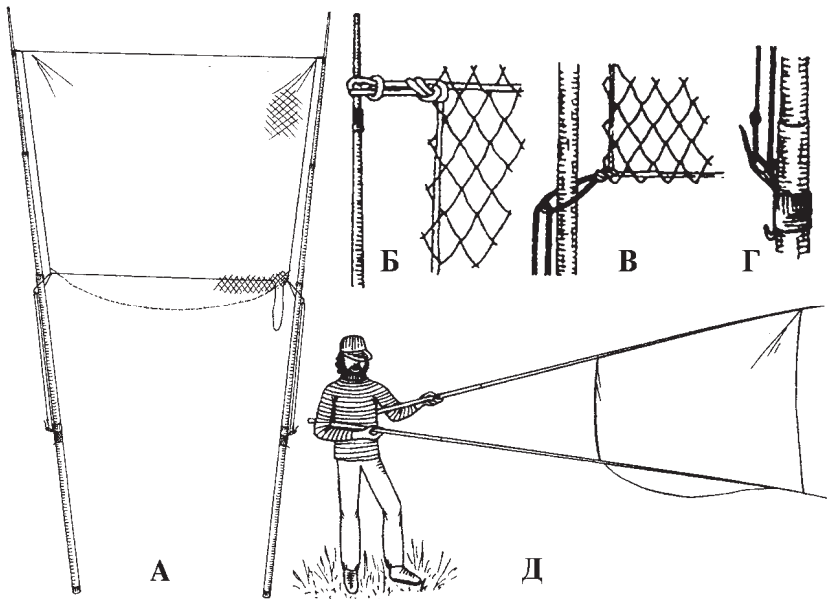
Рис. 3-13. Мобільна пастка. А — загальний вигляд; кріплення до вудлища верхнього (Б) та нижнього (В) країв сітки і гумової стрічки (Г); Д — “стандартний” спосіб тримання пастки (рисунок В. Росіної, за: [6]).
