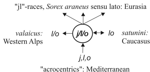
Рис. 3. Вероятная схема базальной радиации надвида Sorex araneus ( sensu lato ) и эволюционный «разлом» кариогруппы " j/l/o " (Zagorodniuk, Khazan, unpubl. data).
