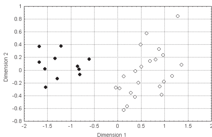
Рис. 1. Краниометрическое сравнение материковых ( minutus , белые значки) и крымских ( dahli , залитые значки) Sorex из группы " minutus ": многомерное шкалирование данных по 11 промерам черепа.
