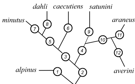
Рис. 4. Схема построения и организации оригинального ключа к определению видов рода Sorex фауны Украины и сопредельных территорий. Узел «5» соответствует надвиду Sorex minutus , узел «10» — надвиду S. araneus .
