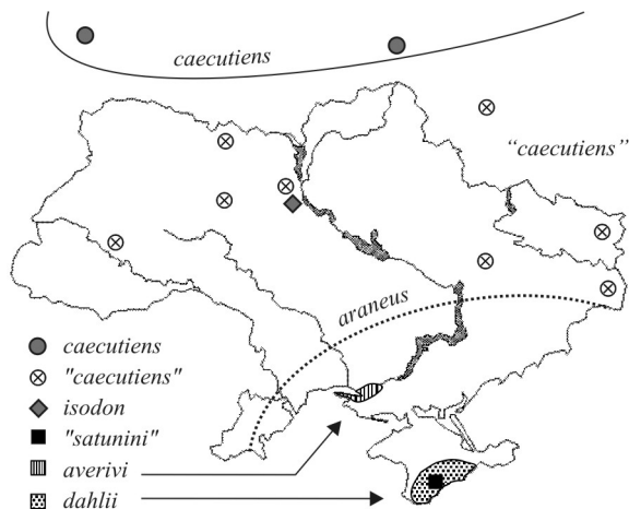
Рис. 6. Места находок «новых» и редких видов землероек в Украине: " caecutiens " (см. текст), " isodon " (Межжерин, 1995), " satunini " (см. текст), araneus и dahli (кол. ЗМКУ и ЦНПМ). Двойной линией отмечена южная граница сплошного распространения бурозубок ( Sorex ).
