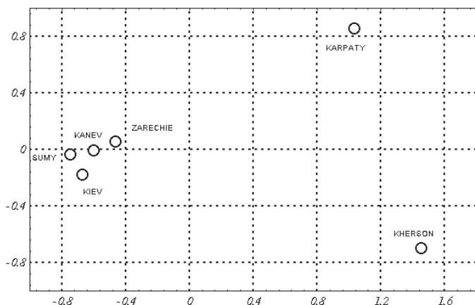
Рис. 2. Положение нижнеднепровской формы averini (выборка «Kherson») в многомерном пространстве среди других географически взаимоудаленных выборок Sorex araneus (по данным из работы В. Межжерина с соавт., 1984).
