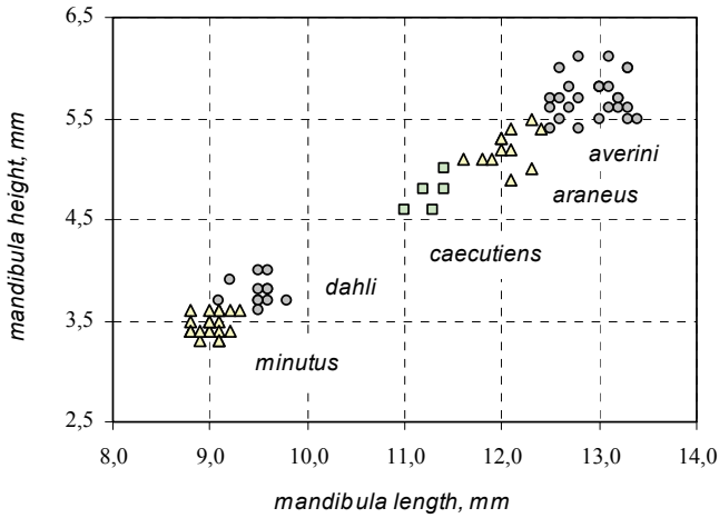
Рис. 5. Размеры нижней челюсти в выборках малых (материковые minutus и крымские dahli ), средних ( caecutiens , Российская Федерация) и обыкновенных ( araneus из Киевской и Черкасской обл. и averini из Херсонской обл.) бурозубок.
