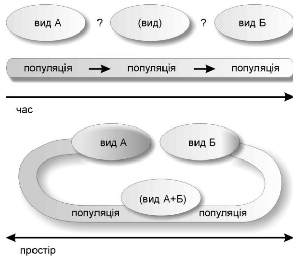
Рис. 2. Співвідношення понять популяція, старий вид (вид А), та новий вид (вид Б) на різних фазах видової диференціації: у часі та у просторі. Вид — це дискретний стабілізований у часі та/або у просторі морфотип; натомість популяція є неперервною у часі і просторі біосистемою.
