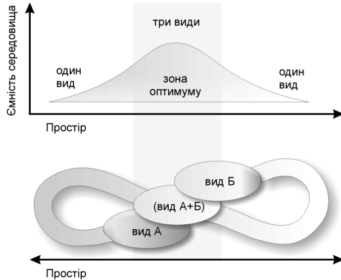
Рис. 3. Модель просторового розподілу роду та його видів: правил А+Б та два його аловици – вид А і вид Б. Зонаю високої таксономічної ємності середовища для цього роду є будь-яка точка простору, проте найімовірніше нею буде типове місцезнаходження правиду. При інвазійному типі формоутворення зона видового багатства роду може не збігатися з його типовою територією.
